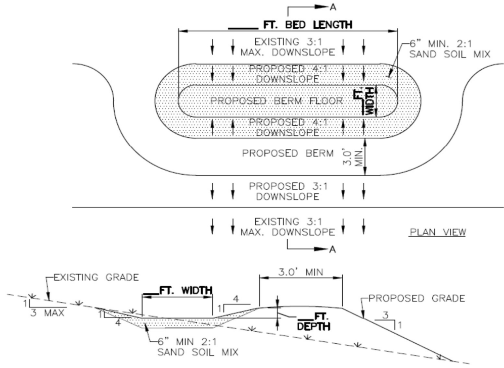
INFILTRATION BERM DETAIL SECTION A-A SCALE: N.T.S.
